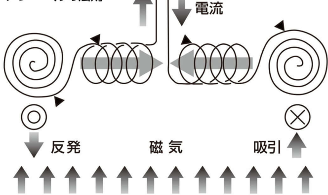
アンペールの法則
